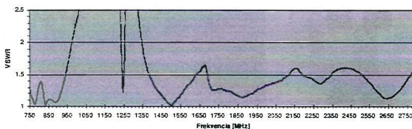
Állóhullám arány
