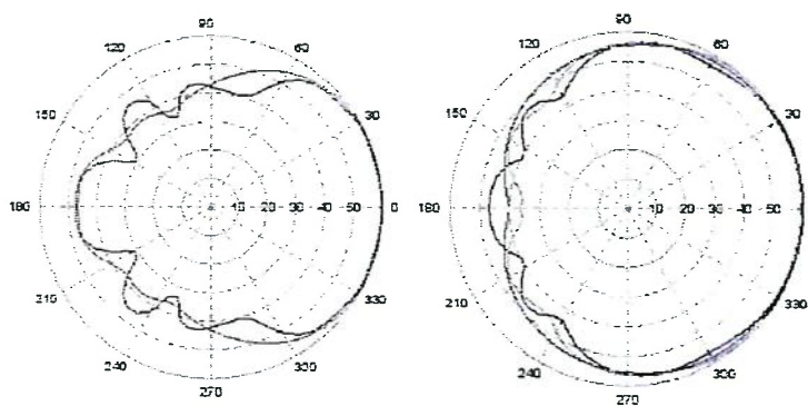
E és H sugárzási karakterisztikák
